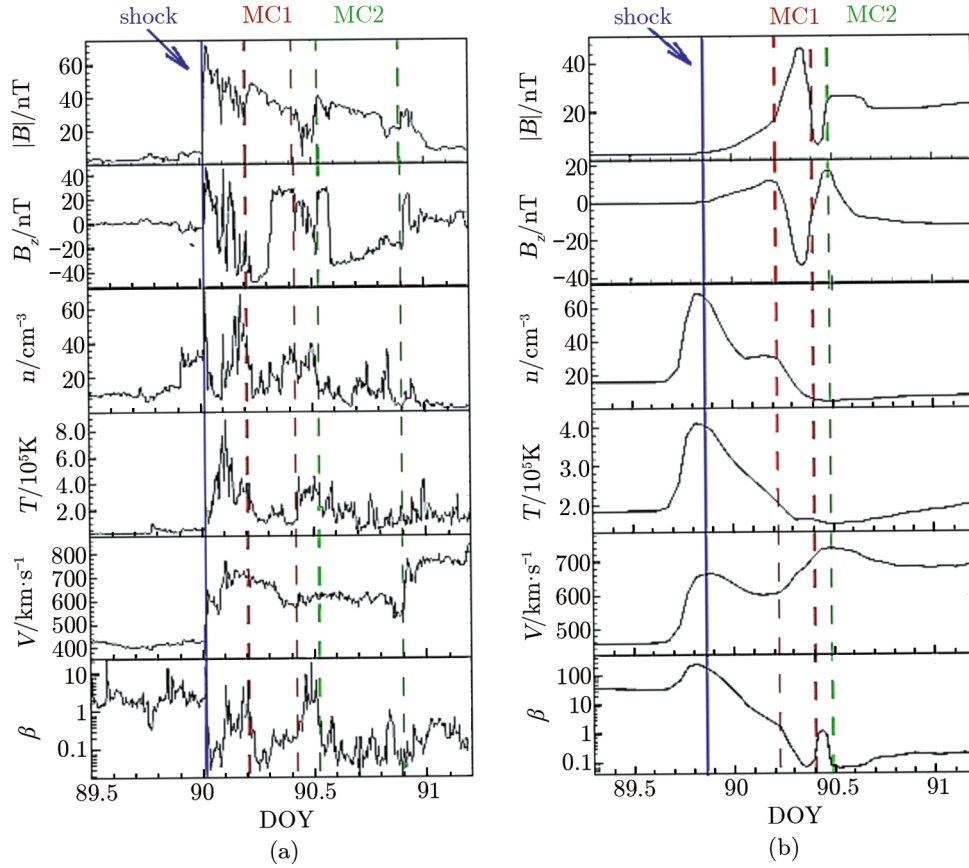
图 12 2001 年 L1 点 ( 213 R_s ) 处磁场和等离子体参数的模拟结果与 ACE 飞船的观测结果对比 [93]
