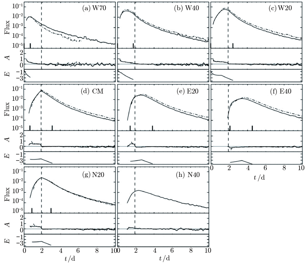
图 7 在有垂直扩散 (实线) 与没有垂直扩散 (虚线) 的情况下, 对比 5 MeV 质子的通量和各向异性 [35]
