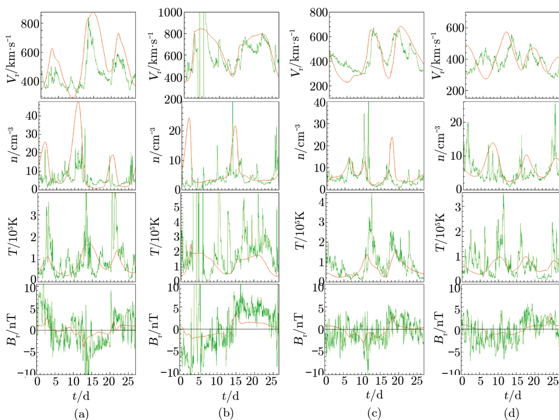
图 11 不同卡林顿周期内的太阳风参数在 1 AU 处的模拟结果与观测结果的对比 [83]
